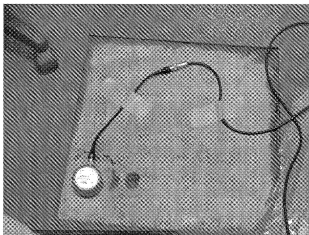
ピックアップ PV-83C (左下部の円筒状のもの)
