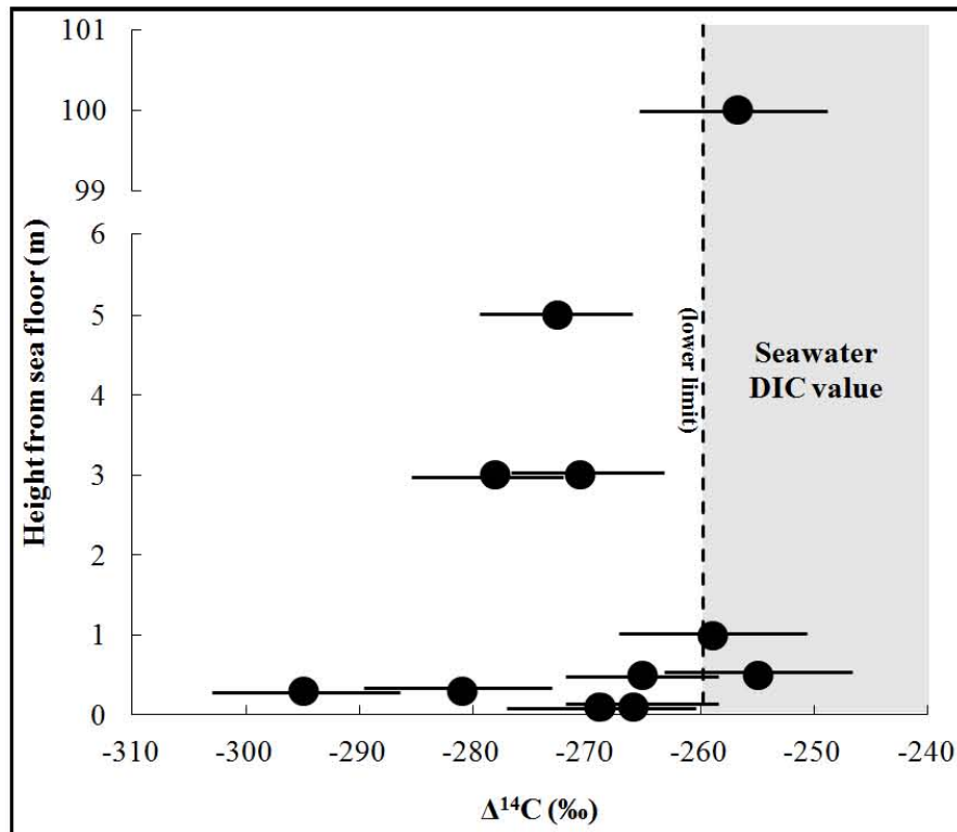
図2. 石灰岩露頭近傍の海水中的の溶存無機炭素の \Delta^{14}\text{C} 値
