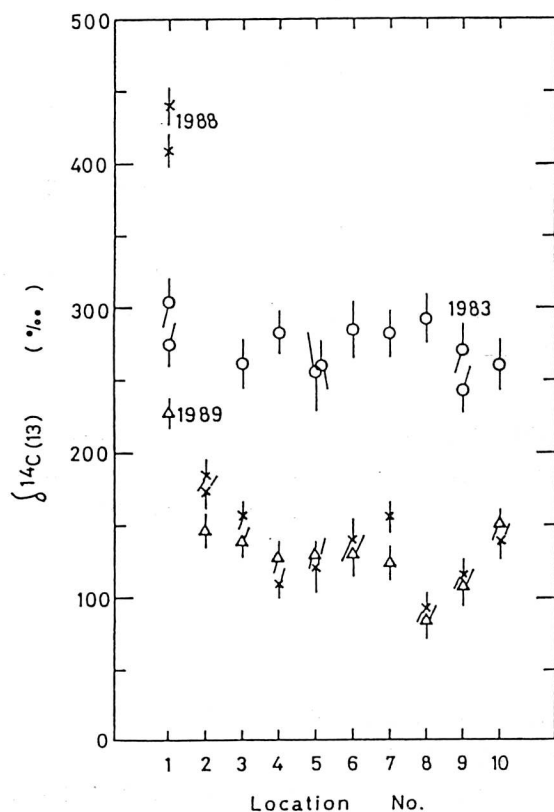
図 2. ^{14}\text{C} 濃度 vs. 松葉試料の採集位置。
