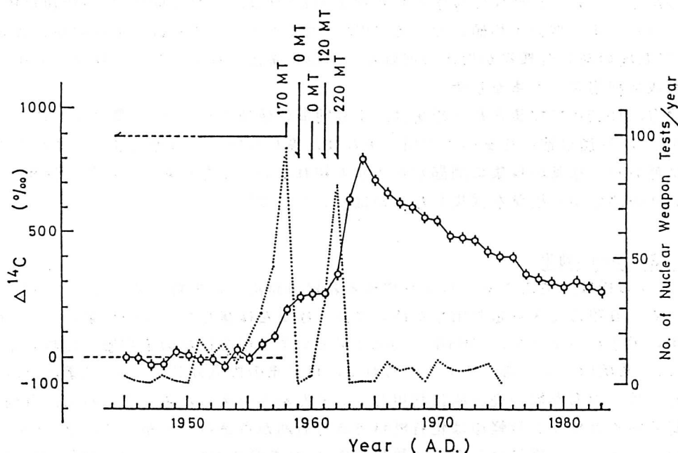
図 3. 木曾ヒノキの年輪の ^{14}\text{C} 濃度の経年変化。
