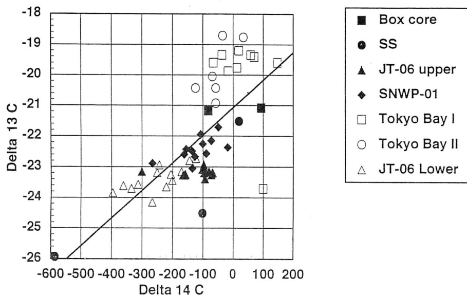
図5 相模湾状海盆における海底堆積物表面泥、懸濁粒子および沈降粒子有機物の \delta^{13}\text{C} および \Delta^{14}\text{C} の相関
