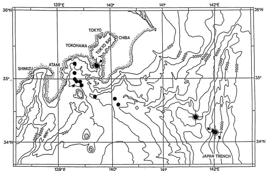
図2 相模湾状海盆における海底堆積物表面泥（●）、懸濁粒子（▲）および沈降粒子採集点（⊙）
