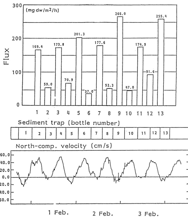
図3 東京湾口の時系列型セディメントトラップによる沈降粒子束と海水流動の変動
