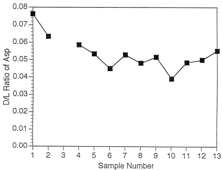
図4 東京湾口の時系列型セディメントトラップ試料におけるアミノ酸D/L値の変動
