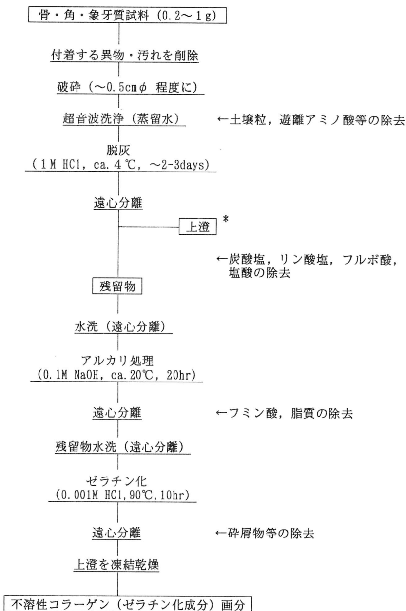
図1 骨に残存する酸不溶性コラーゲンの抽出操作 不溶性画分の回収を良くするため、脱灰からゼラチン化までの 操作は同一の試験管（スクリーキャップ付き遠心沈澱管）内で行う。
