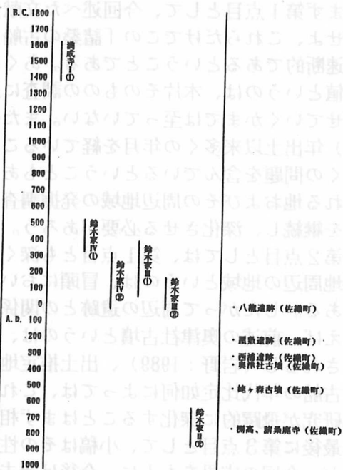
図5 「諸桑の古船」 14 C年代測定結果
