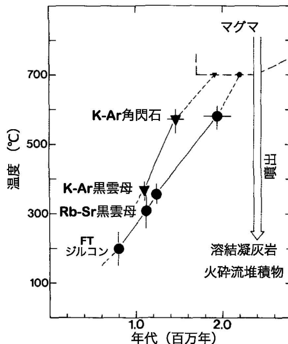
図2. 滝谷花こう岩類およびそれに関連する火成岩類の冷却過程 (Harayama, 1992).
